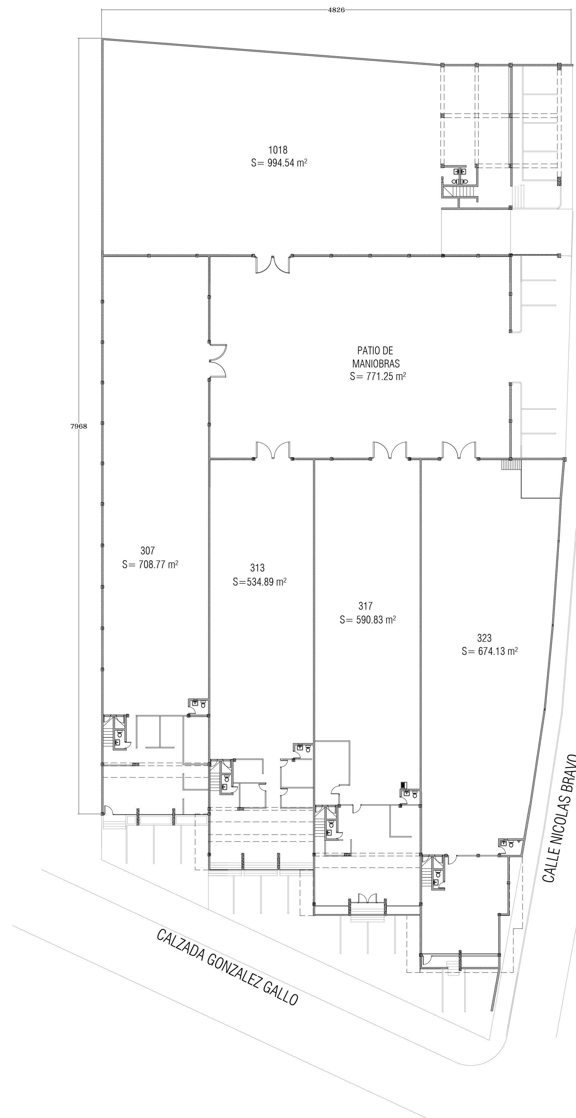
PLANTA BAJA (PLANO GENERAL) ESC. 1:200 [cm]
